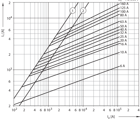
Omezovací charakteristika
