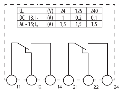
3NP1933-1GB30 3NP1933-1GB50
