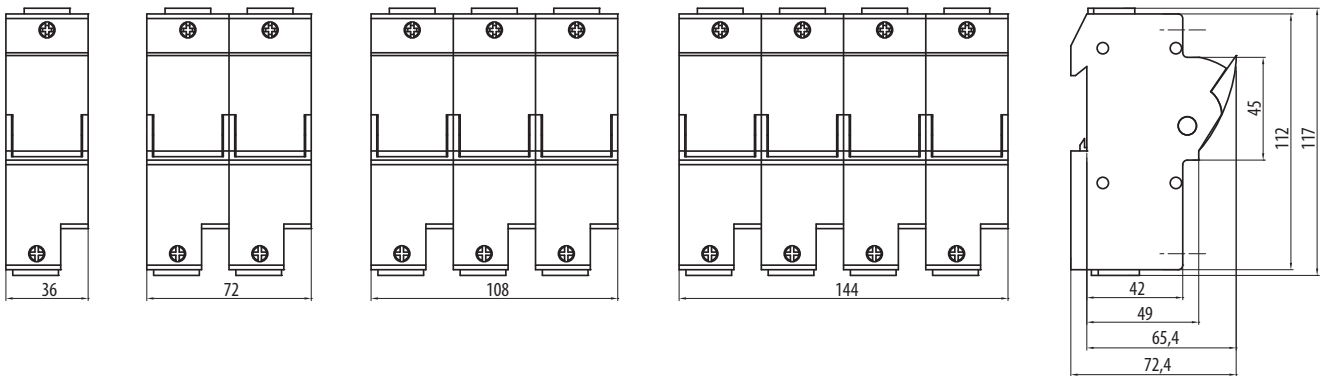
OPVP22-1N OPVP22-2..
