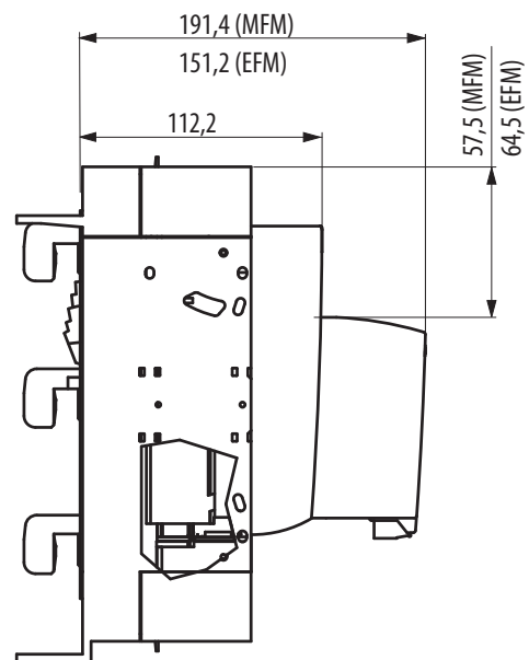
3NP113.-1BC..
