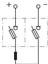
Jednólové zapojení dvou jednólových odpínačů pro DC aplikace, viz Kategorie užítí
