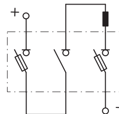
Dvóvólové zapojení třípólového odpínače pro DC aplikace, viz Kategorie užítí
