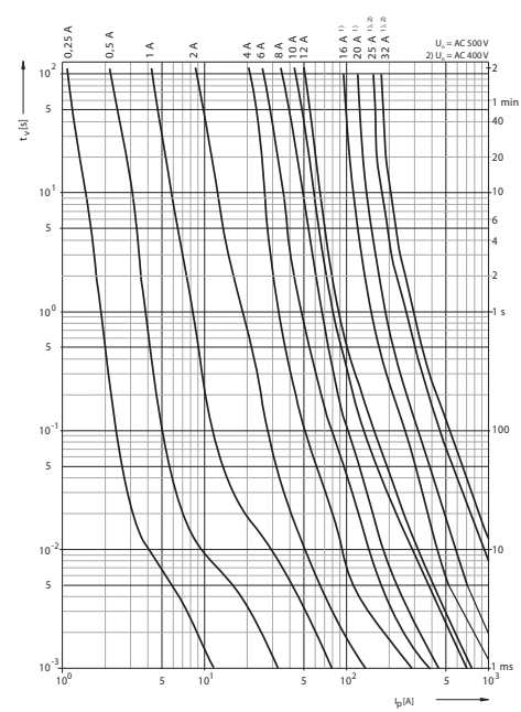
Tavná ampérsekundová charakteristika PVA10, PV10 1) aM
