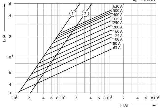
Omezovací charakteristika
