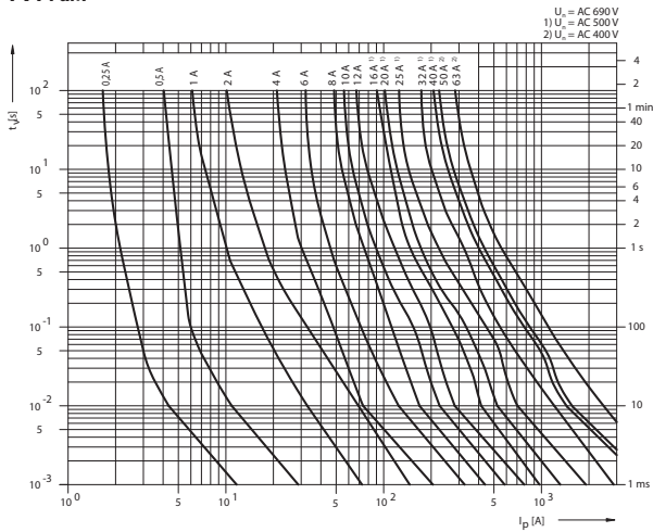
Tavná ampérsekundová charakteristika PV14 aM
