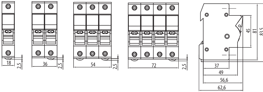
OPVP10-1N OPVP10-2..
