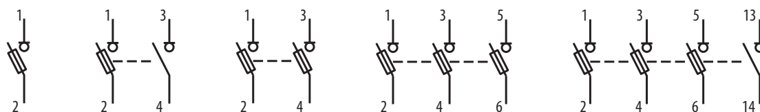
OPVP..-1
