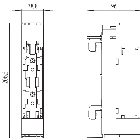
3NP1921-1EE10
