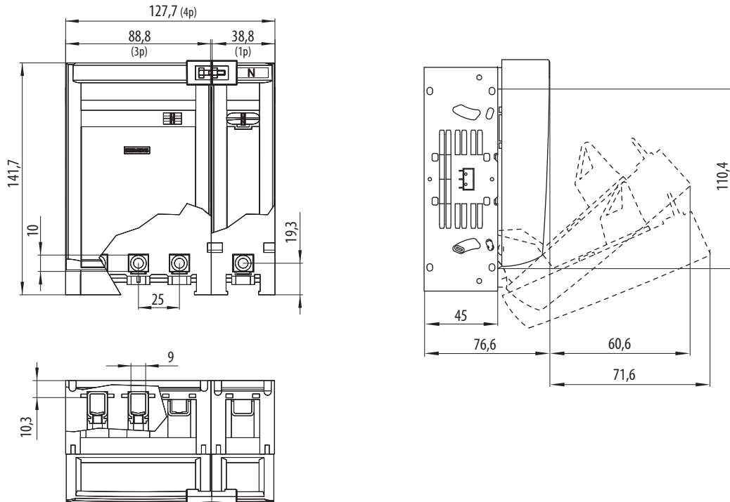
3NP112.-1CA20
