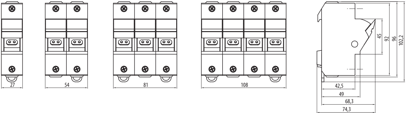
OPVP14-1N OPVP14-2..
