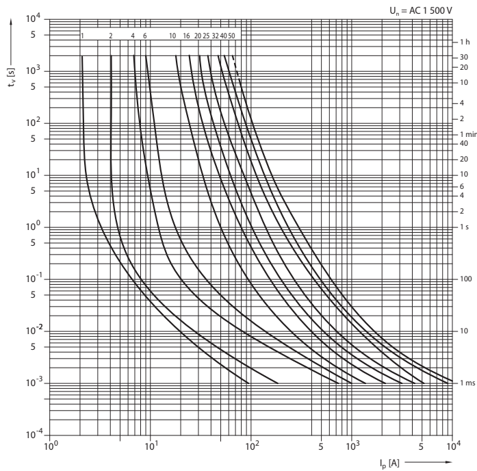
Tavná ampérekundová charakteristika PT22
