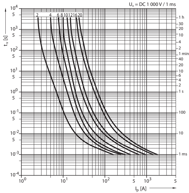
Tavná ampérekundová charakteristika PC10 gPV
