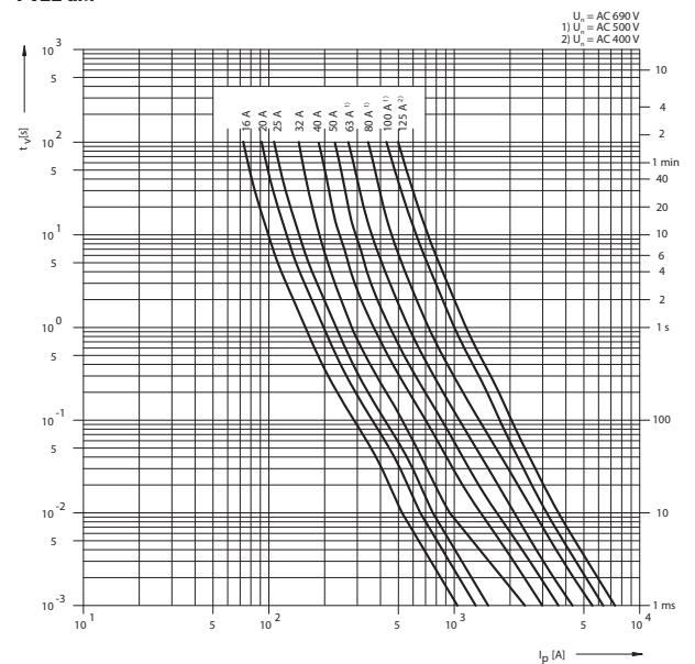
Tavná ampérsekundová charakteristika PV22 aM
