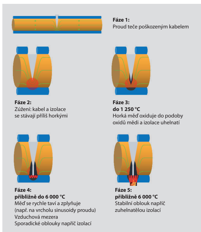
Vypuknutí požáru v důsledku sériových oblouků
