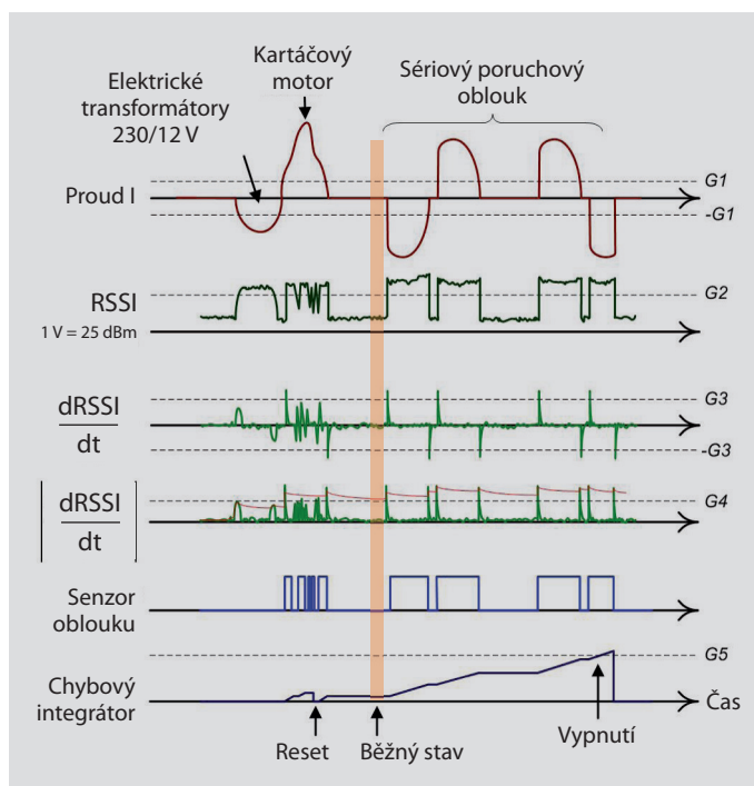
Vyhodnocení signálu při detekci sériového chybového oblouku
