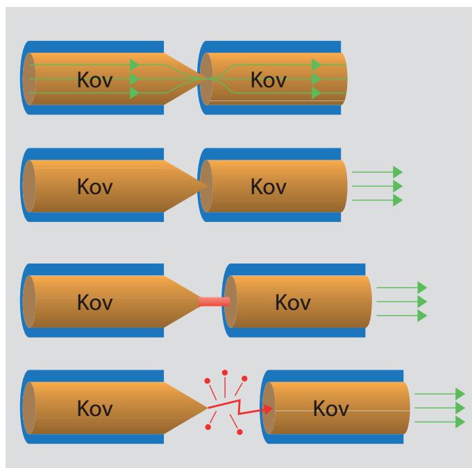
Oblouk na kontaktech
