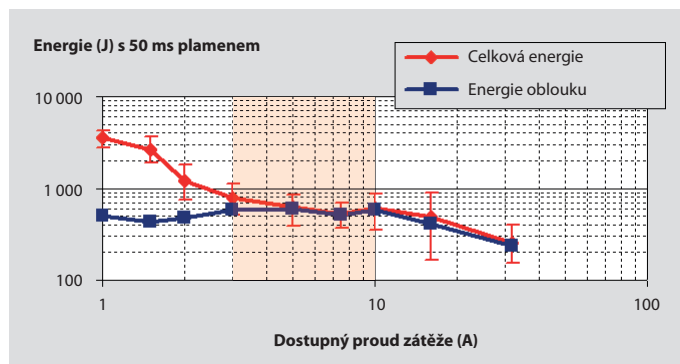
Energie významného plamene v závislosti na proudu zátěže
