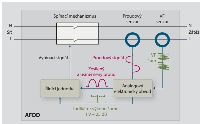
Základní konstrukce AFDD
