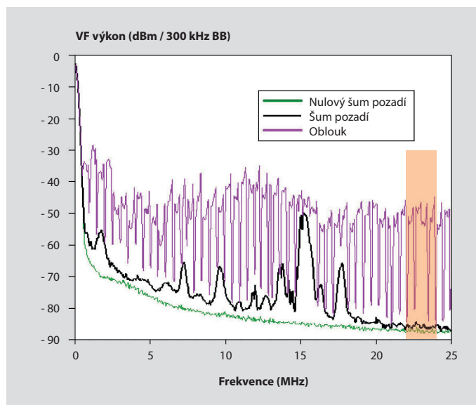
VF šum (šum pozadí a oblouků)
