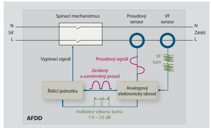
Základní konstrukce AFDD
