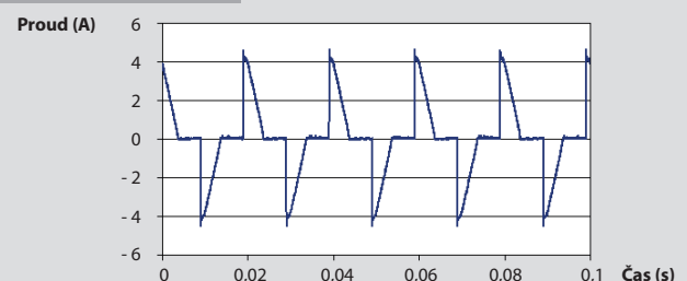
Příklady elektrických zátěží s VF signály
