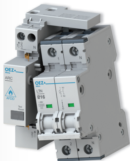
Sestava s jističem
