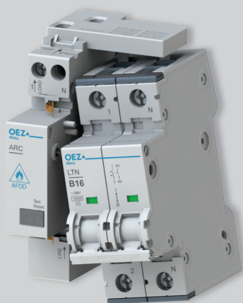
ARC-16-1N-M3 + LTN-16B-1N
