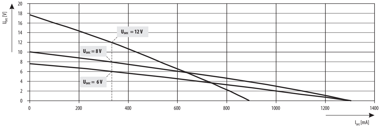
Zatěžovací charakteristika UNZ-10T-., UNZR-10T-X024 - AC výstup
